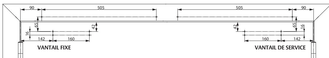
Configuration de montage porte côté charnières
