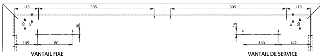
Configuration de montage porte côté opposé aux charnières
