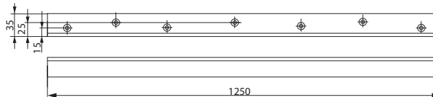
Support équerre A117 appui central pour montage du bras à glissière G464 côté opposé aux charnières.
