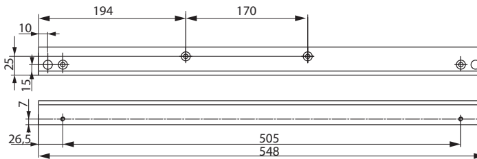
Support équerre A116 pour montage du bras à glissière G464 côté opposé aux charnières.
